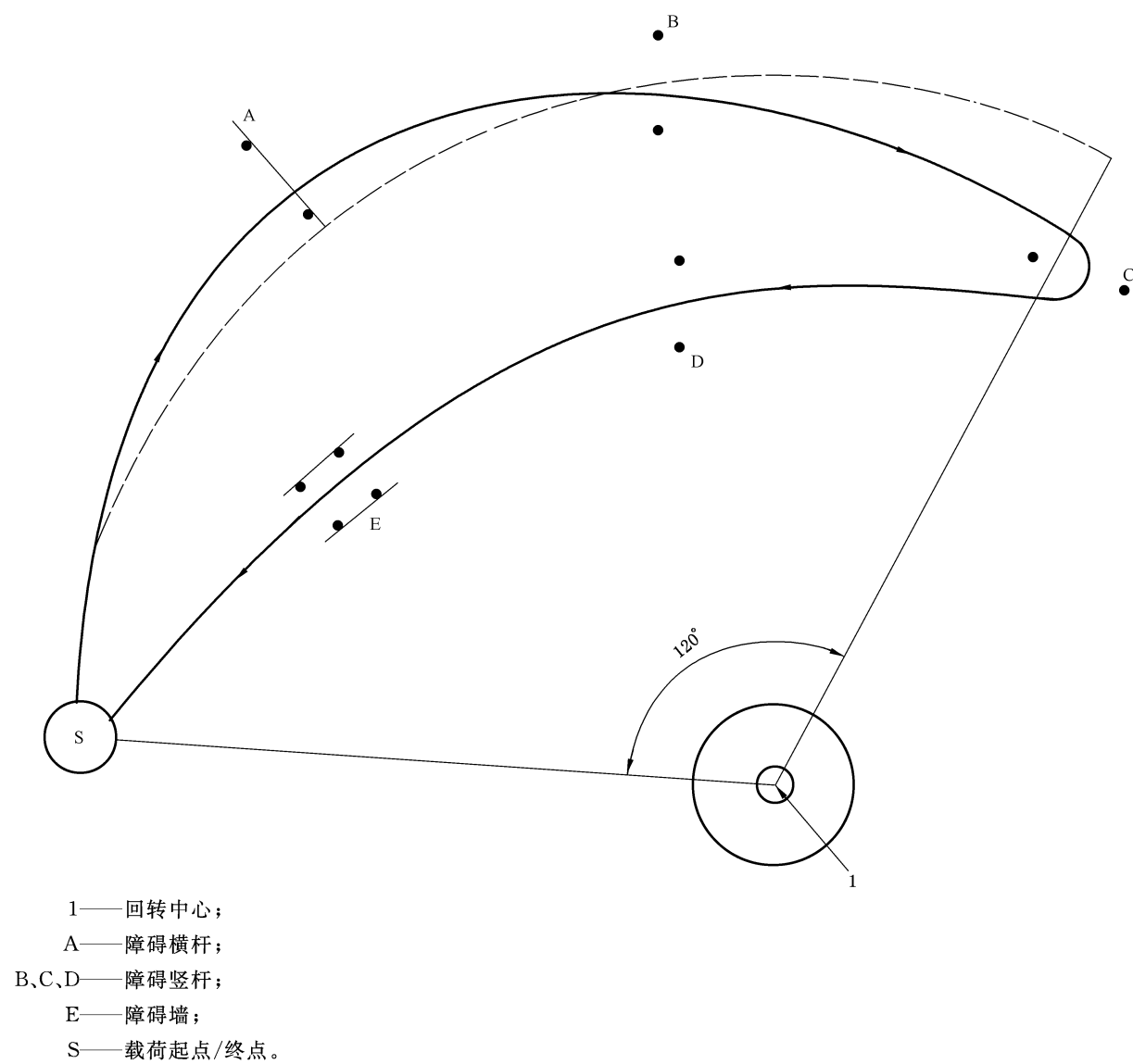
图 C.3 臂架起重机和流动式起重机的测试线路
